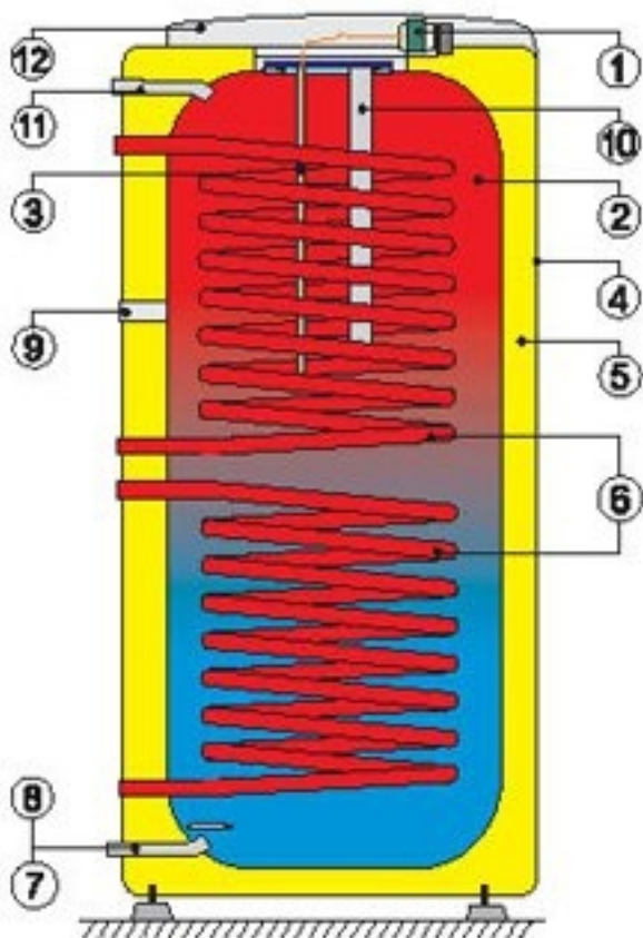
Схема конструкции водонагревателя
