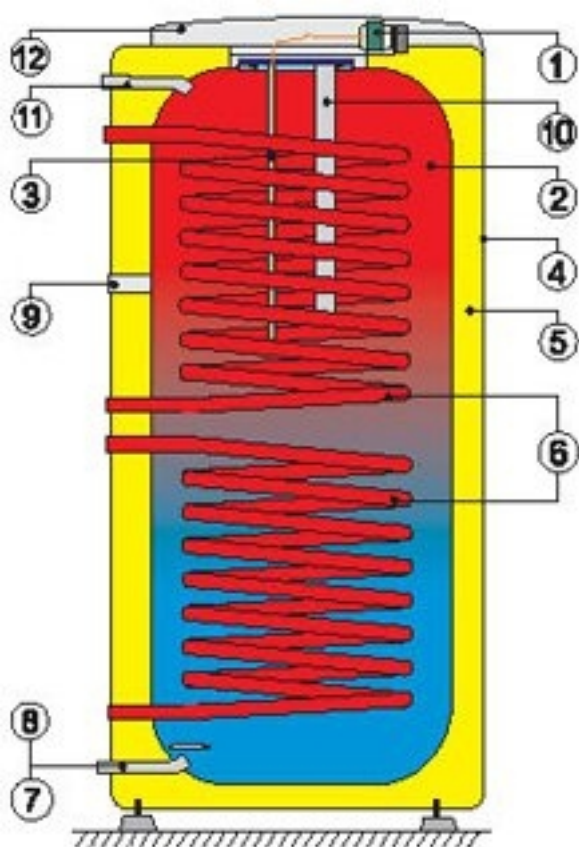
Схема конструкции водонагревателя ОКС 250 NTRR
