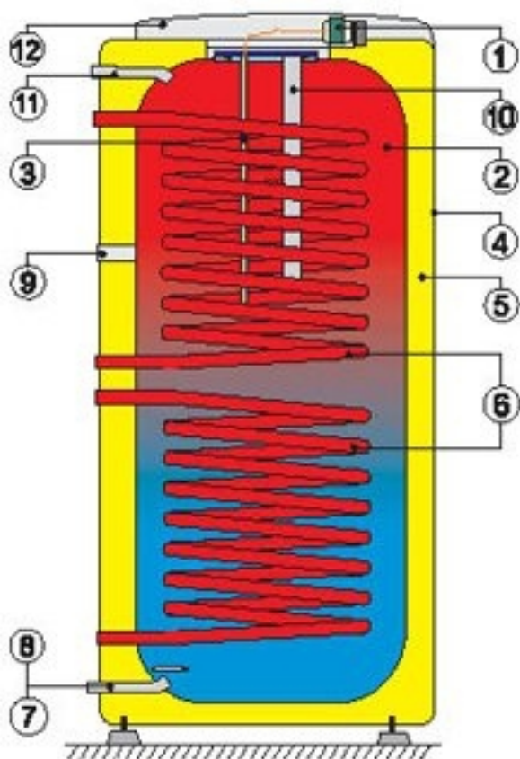
Схема конструкции водонагревателя ОКС 250 NTRR
