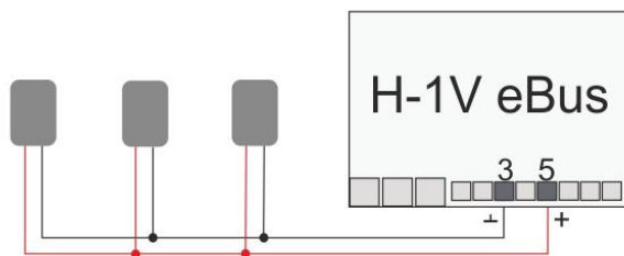
Датчик DS18S20
