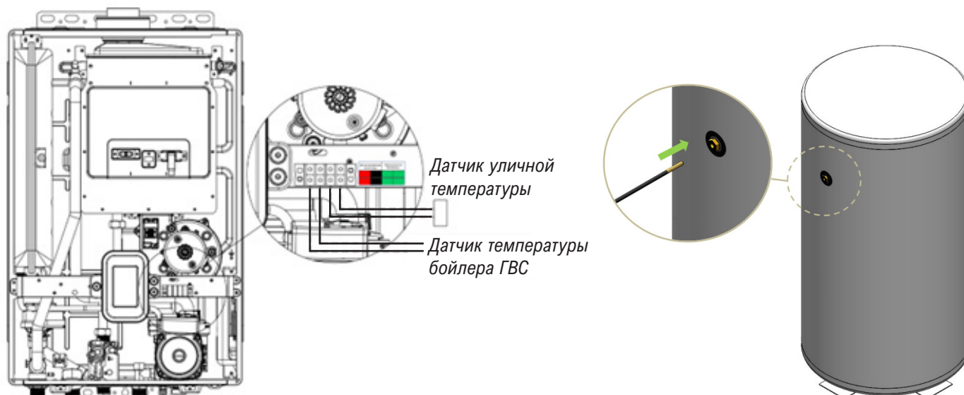
Рисунок 14. Подключение датчика температуры ГВС в бойлере.
