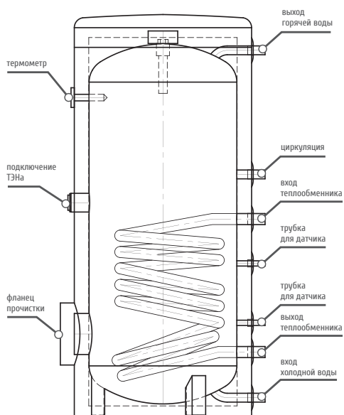
БОЙЛЕРЫ С ОДИМ ТЕПЛООБМЕННИКОМ
