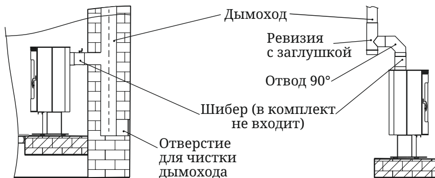
а) к стационарному дымоходу из кирпича
