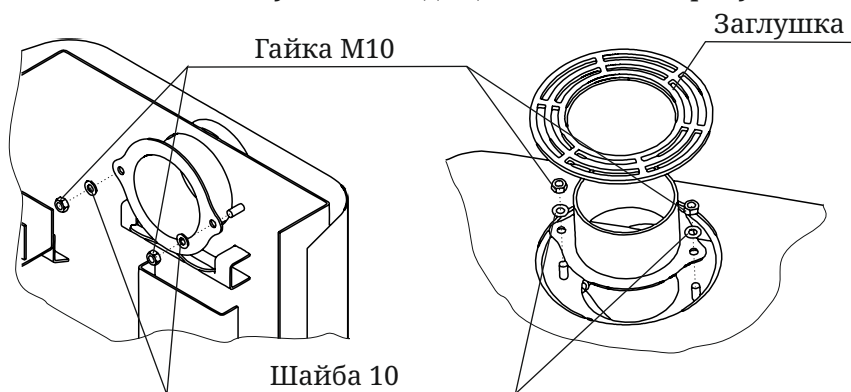
Рисунок 7. Схема установки коннектора дымохода
