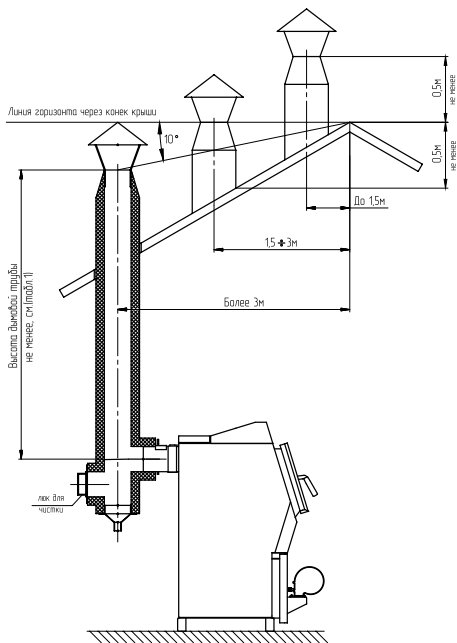
Рис.5 Варианты установки дымовой трубы
