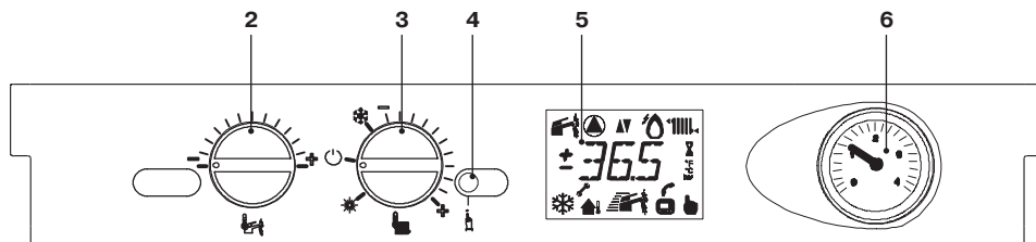
Рисунок 1.3. Панель управления
