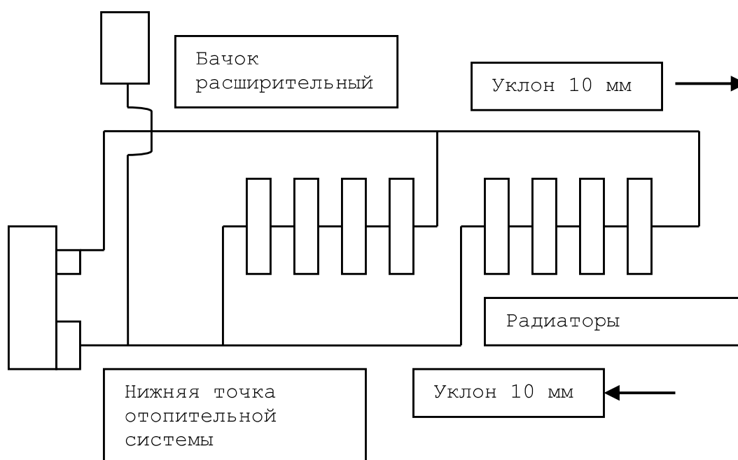
Рис. 1. Схема монтажа системы отопления открытого типа.
