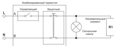
Рис. 8. Схема электрическая для моделей E-series, OPPro, EGO, OPPro+
