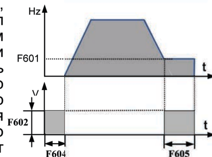
Рис 5-9 Торможение
