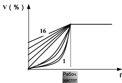
Рис 5-3 Крутящего момента
