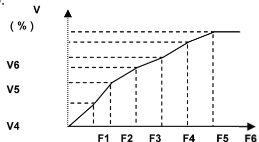
Рис 5-4 Многоточечная
