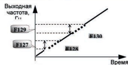
Рис 5-2 Пропуск частоты
