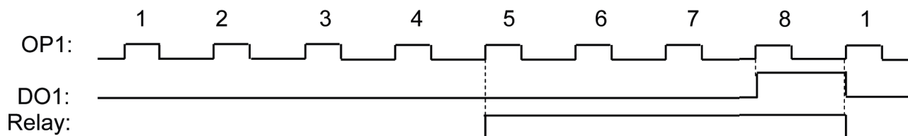
Рис 5-6
