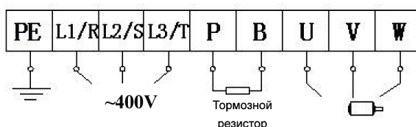
Силовой терминал
