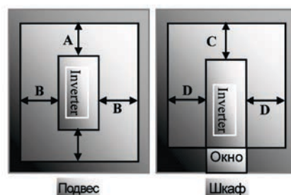
Рис.3-1 Установка
