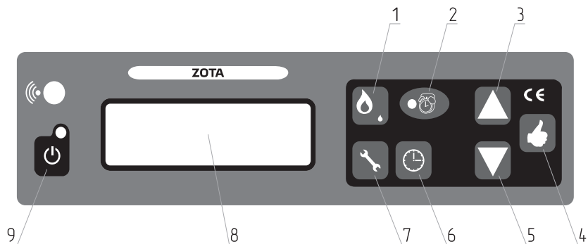
Рис.7 Устройство панели управления
