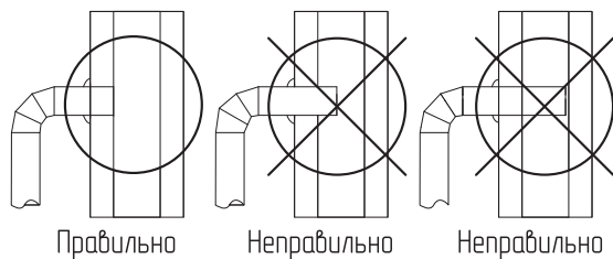
Рис.3 Подключение дымоотводящей трубы к кирпичному дымоходу
