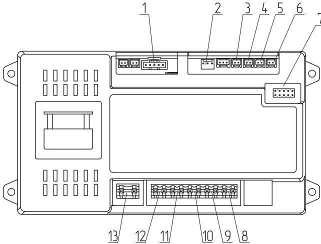
Рис.6 Подключение панели управления
