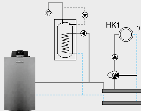
*) Нагревательный контур или контур котла по выбору.
