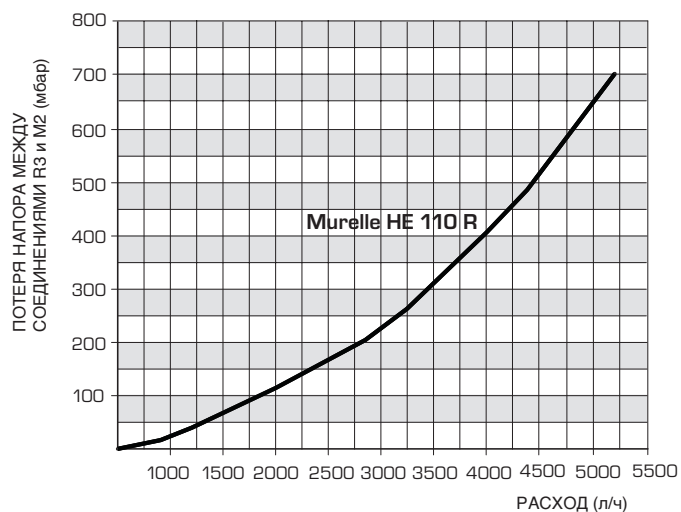
КРИВАЯ ПОТЕРЯ НАПОРА/РАСХОДА МЕЖДУ СОЕДИНЕНИЯМИ R3 и M2
